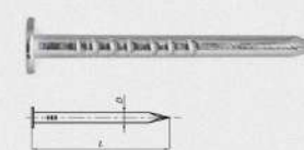
Гвозди цинковые
