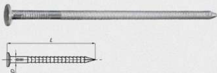
Гвозди ершковые
